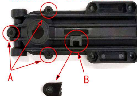
CA3057D テールプーリーケース(R) 『改造後』
